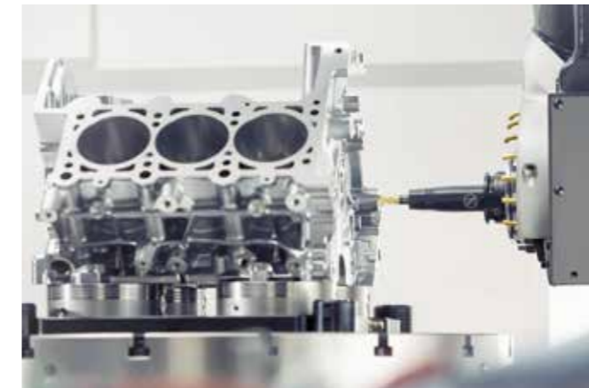
Lavorazione di una testata cilindro motore TENDO Slim 4ax
